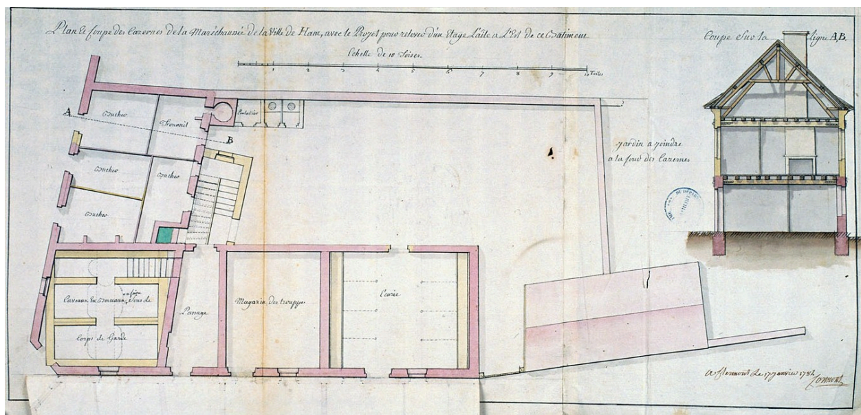
Plan [du rez-de-chaussée] et coupe des casernes de la maréchaussée de la ville de Ham, avec le projet pour relever d'un étage l'aile à l'est de ce bâtiment, dessin, par Cormont, 1784 (AD Somme ; 1C_CP_1641/24).
