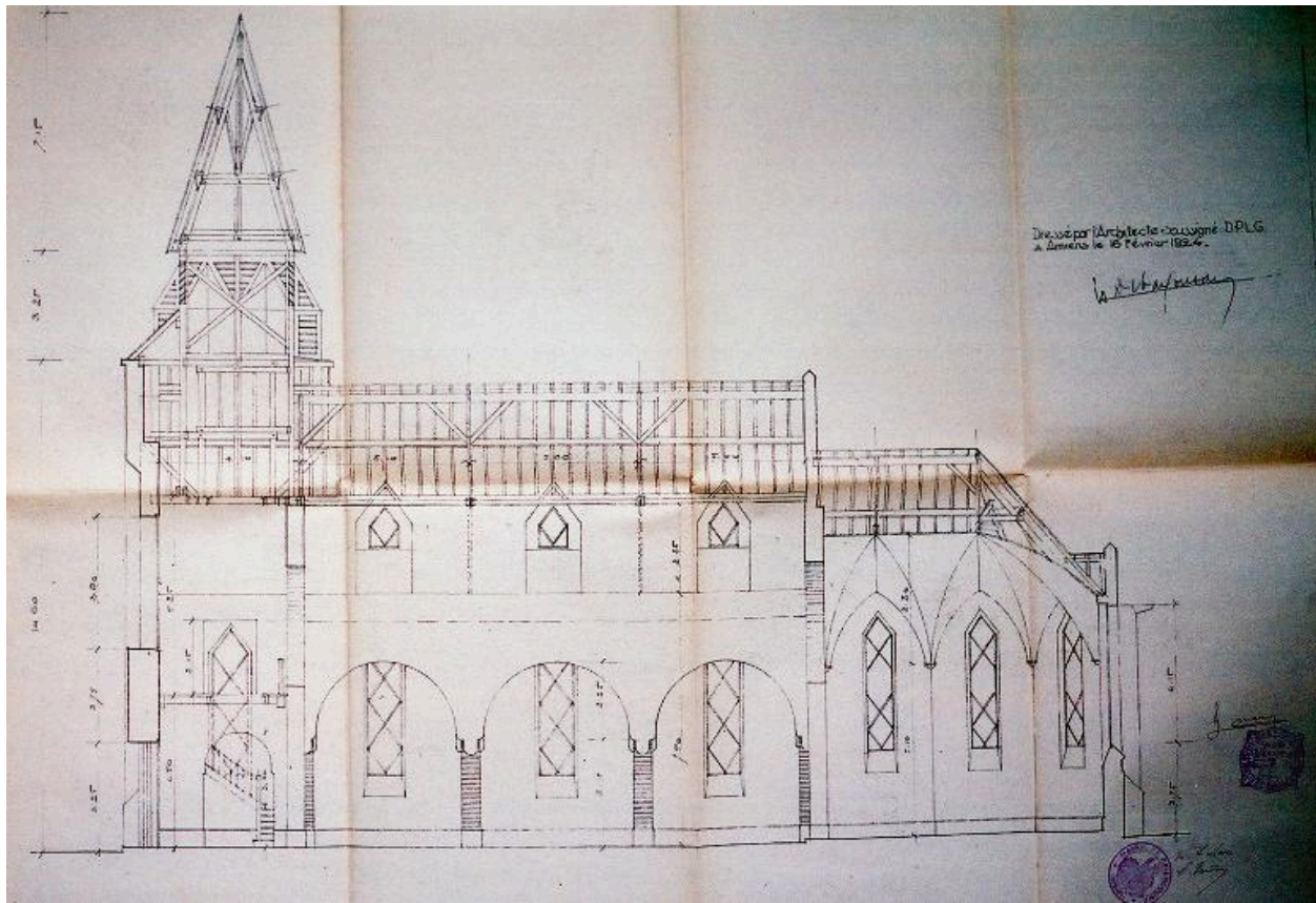
Projet de reconstruction de l'église : coupe longitudinale, Jacques Debat-Ponan (architecte), 16 février 1924 (AD Somme ; 99 O 1468).
