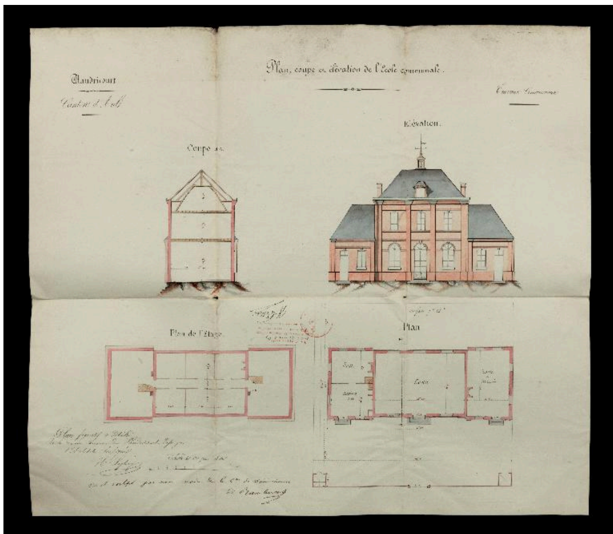
Plan, coupe et élévation de l'école et mairie, Lephey architecte, 1862 (AD Somme ; 99 O 3660).
