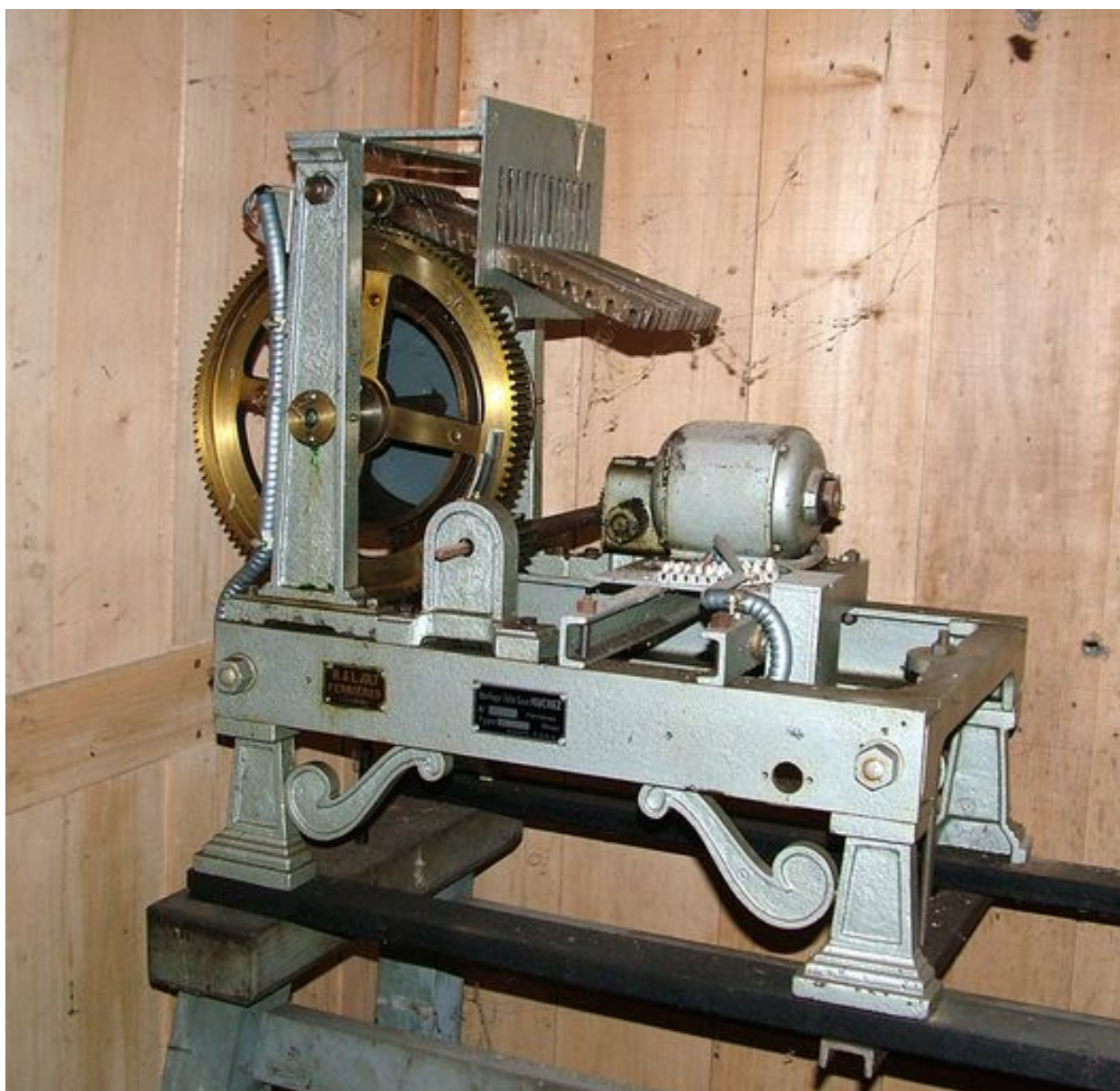
Mécanisme de cloches par M. & L. Joly et Horloge Télé. Sect. Huchez, à Ferrières (Oise), vers 1929.
