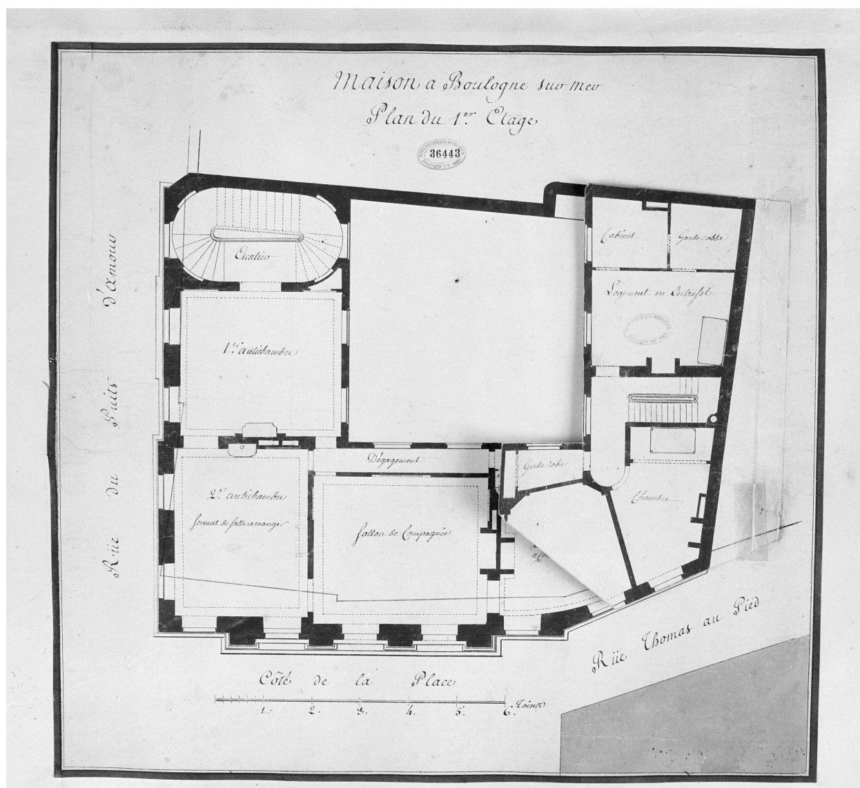
Plan du premier étage. B.M. Boulogne-sur-Mer, 13e portefeuille, fol. 14.
