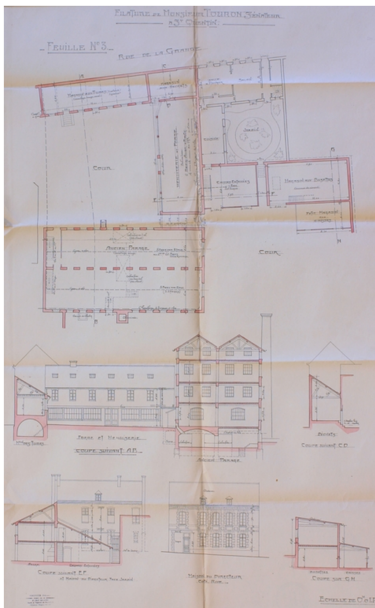
Plan des anciens ateliers de parage (3e quart 19e siècle ?) et ateliers annexes, par Nalet : état en 1914 (AD Aisne).
