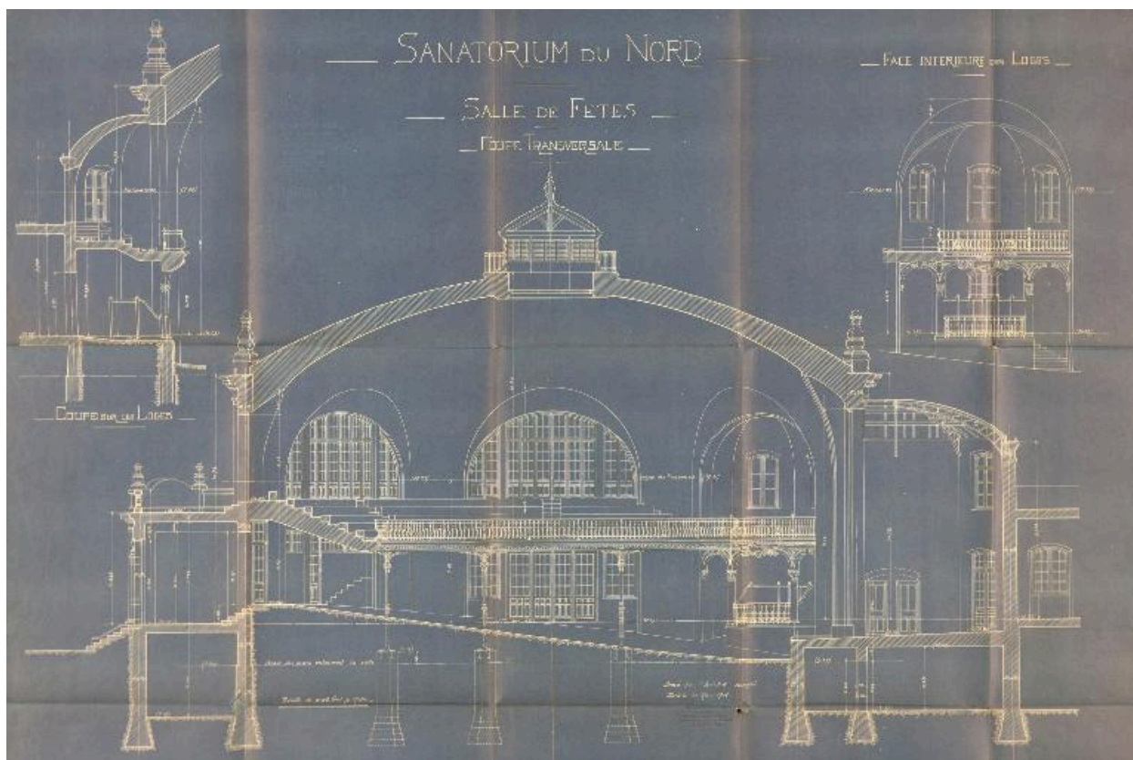
Salle des fêtes, coupe transversale, datée du 20 mars 1906 (IFA).
