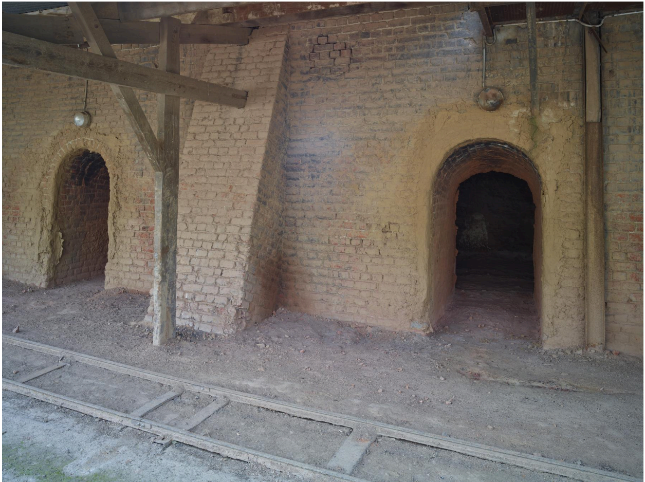
Four Hoffmann. Accès de chargement/déchargement des briques.
