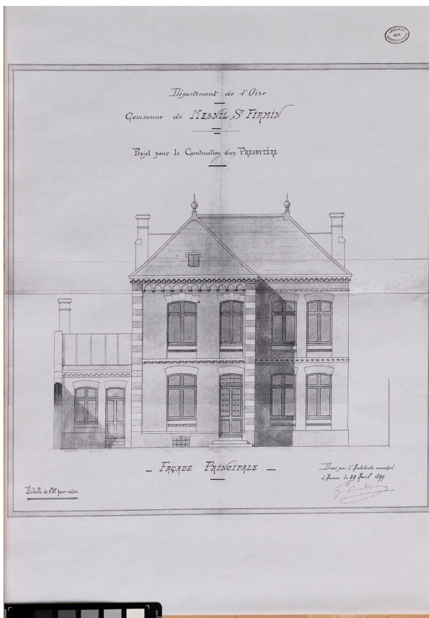
Le Mesnil-Saint-Firmin (Oise). Plan en élévation du presbytère (façade sur rue), Georges Antoine, 1899 (AD Oise).
