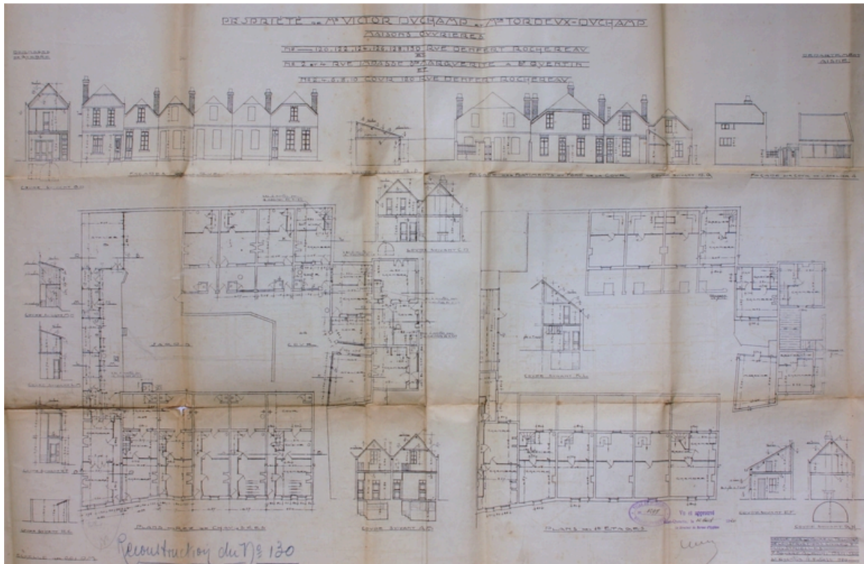
Les plans de la cour Corbizet, Bureau Technique de Constructions Civiles et Industrielles, 1920 (AC Saint-Quentin).
