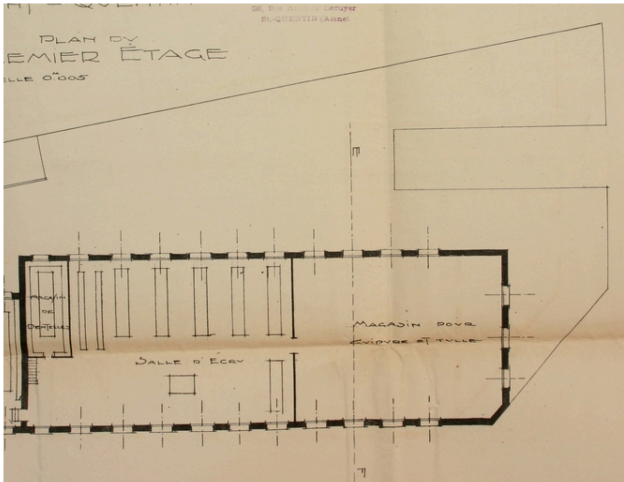
Plan du premier étage de l'usine Trocmé à la veille de la Première Guerre mondiale dressé après 1919 par Chauquet, Navile et Christol. Détail de magasins et de la salle d'écrue (AD Aisne).
