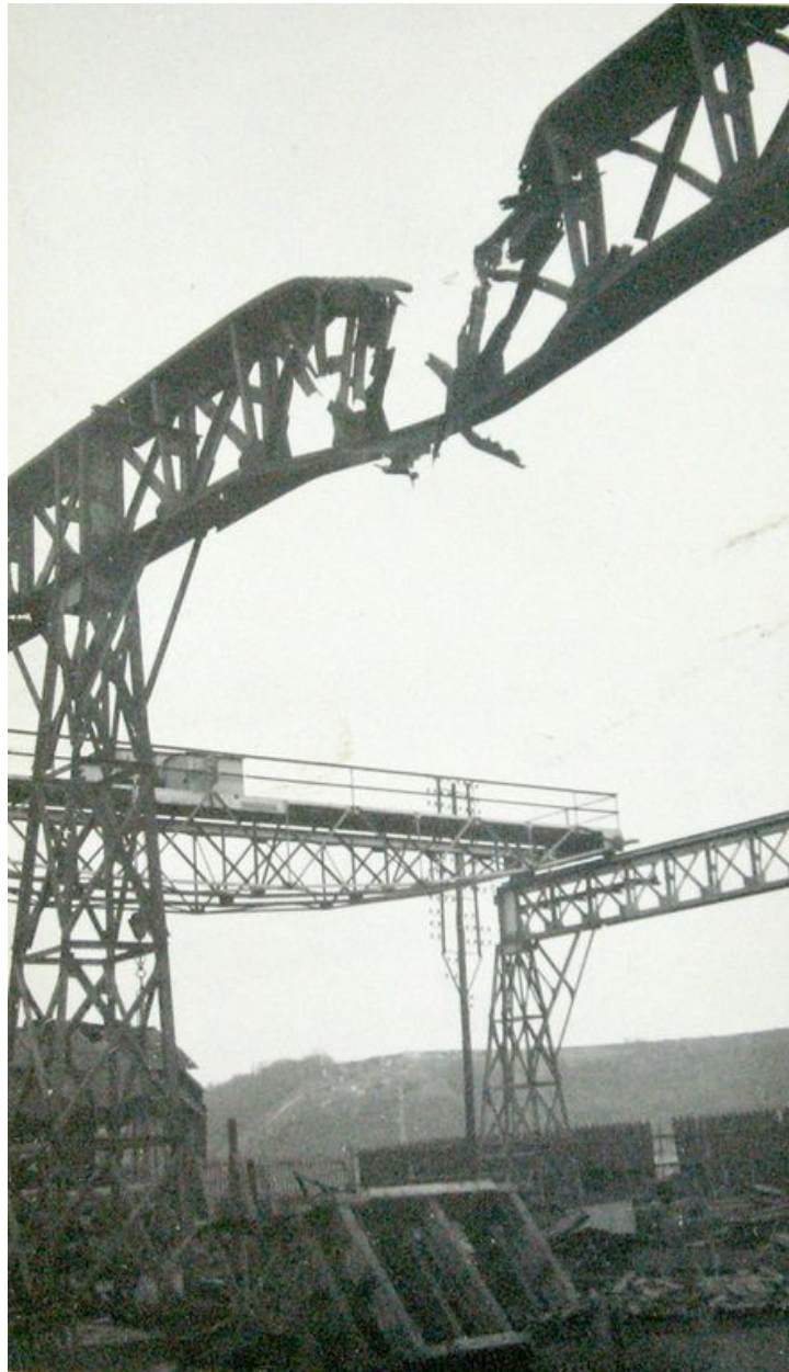
Poutre du chemin de roulement, état après les bombardements de 1944 (AD Oise ; 617W18128).
