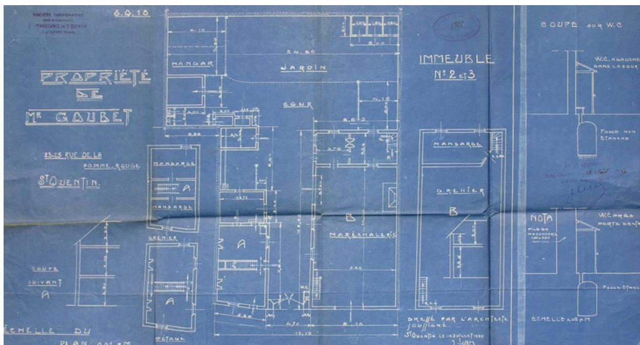
Plan de reconstruction des ateliers et logement de M. Goubet, 1920 (AC Saint-Quentin).
