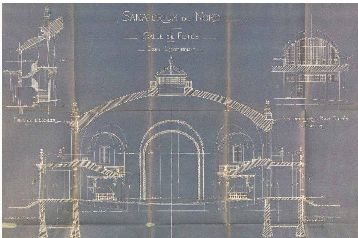
Salle des fêtes, coupe longitudinale, datée du 20 mars 1906 (IFA).
