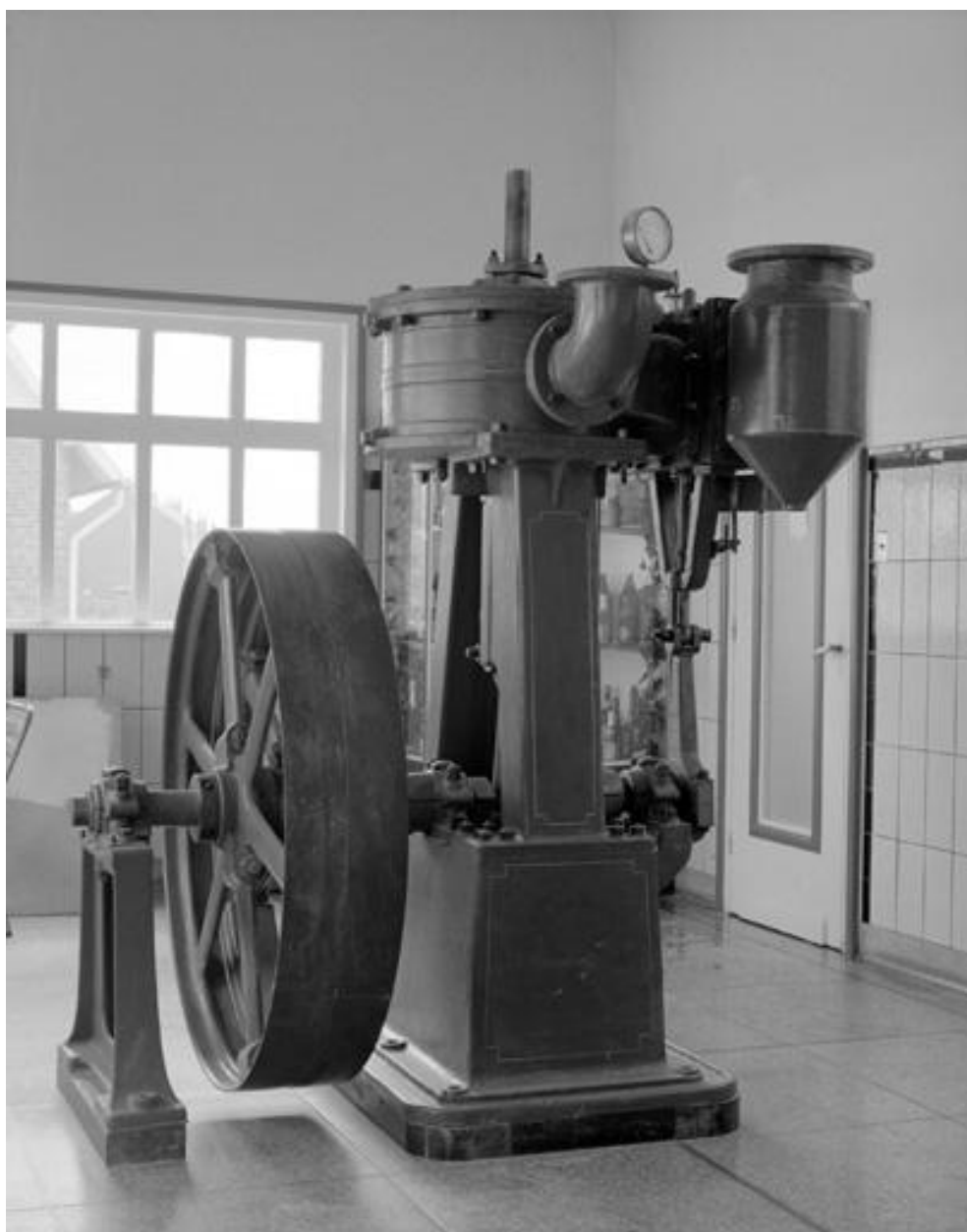
Pompe à vide à membrane. Atelier de construction Seck Frères (Dresde) : vue postérieure.
