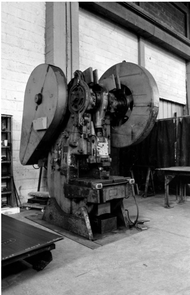
CLAIROIX. Usine d'emboutissage Gantois. Machine de production.
