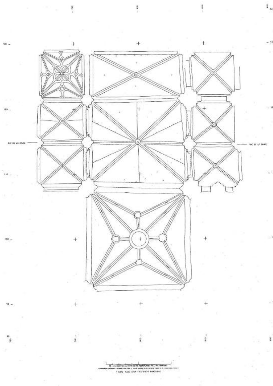
Plan du voûtement de la croisée et du bras nord du transept : restitution photogrammétrique.
