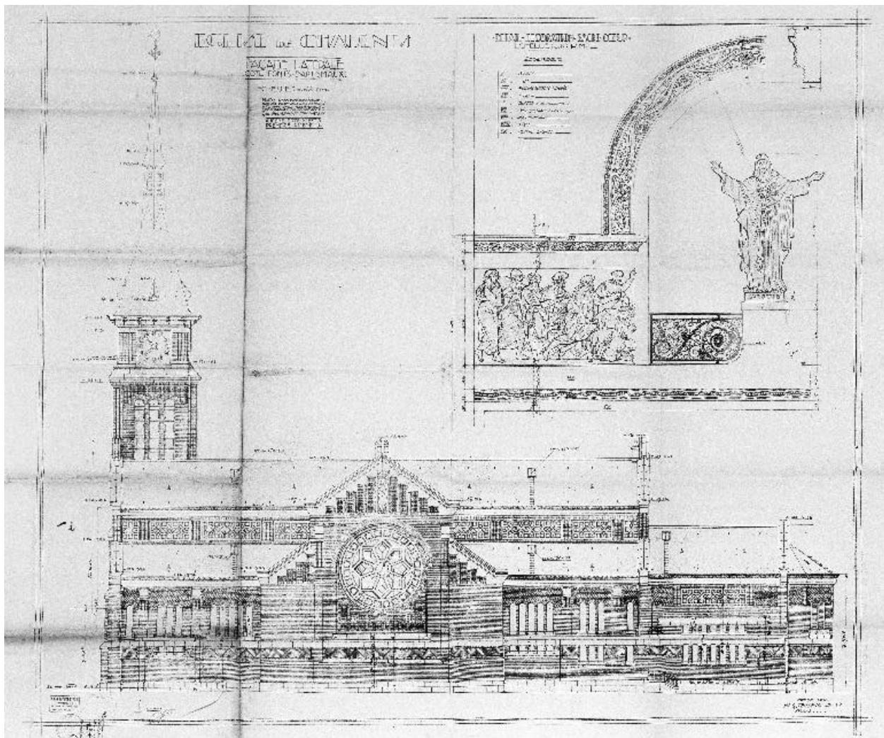
Eglise de Chaulnes [projet de reconstruction]. Façade latérale et fonts baptismaux, tirage du plan de Teisseire arch. et Cie, juin 1928 (AD Somme).
