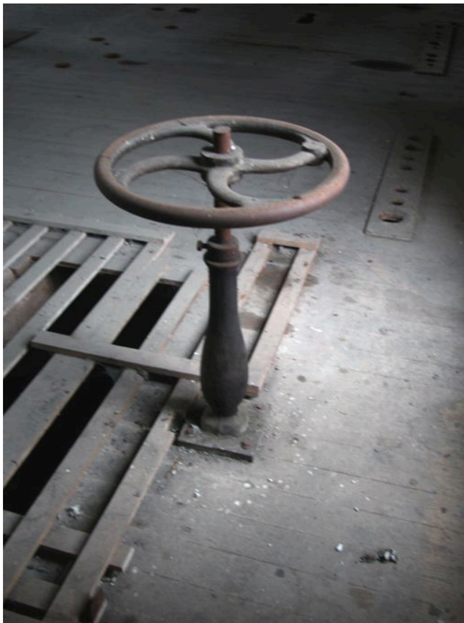
Intérieur du premier étage, détail du volant de commande d'ouverture de la vanne mouloire.
