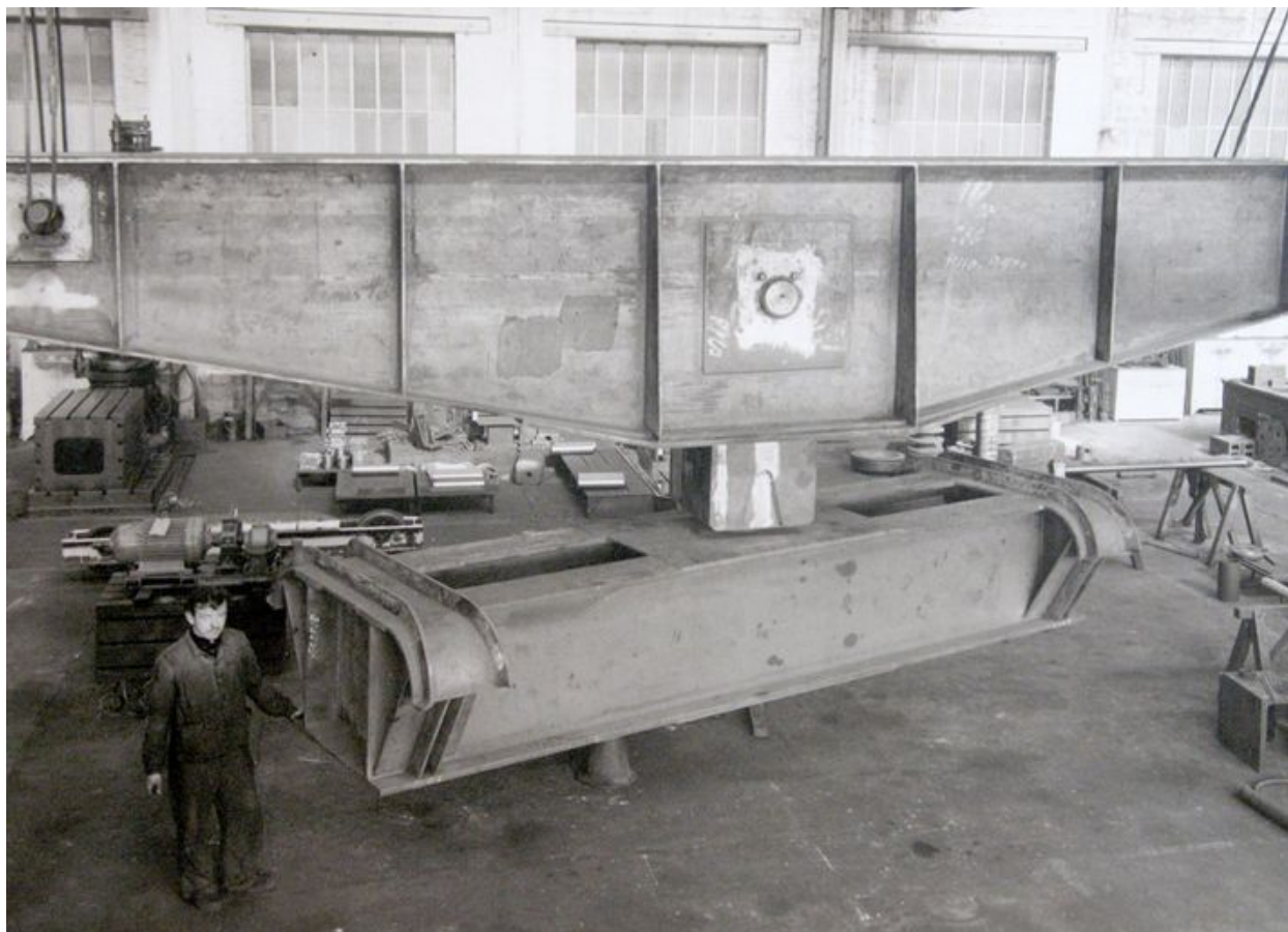
Poutre de jumelage et palonnier de 280 tonnes construits pour l'usine EDF de Vaires-sur-Marne en Seine et Marne, 1961 (AP).
