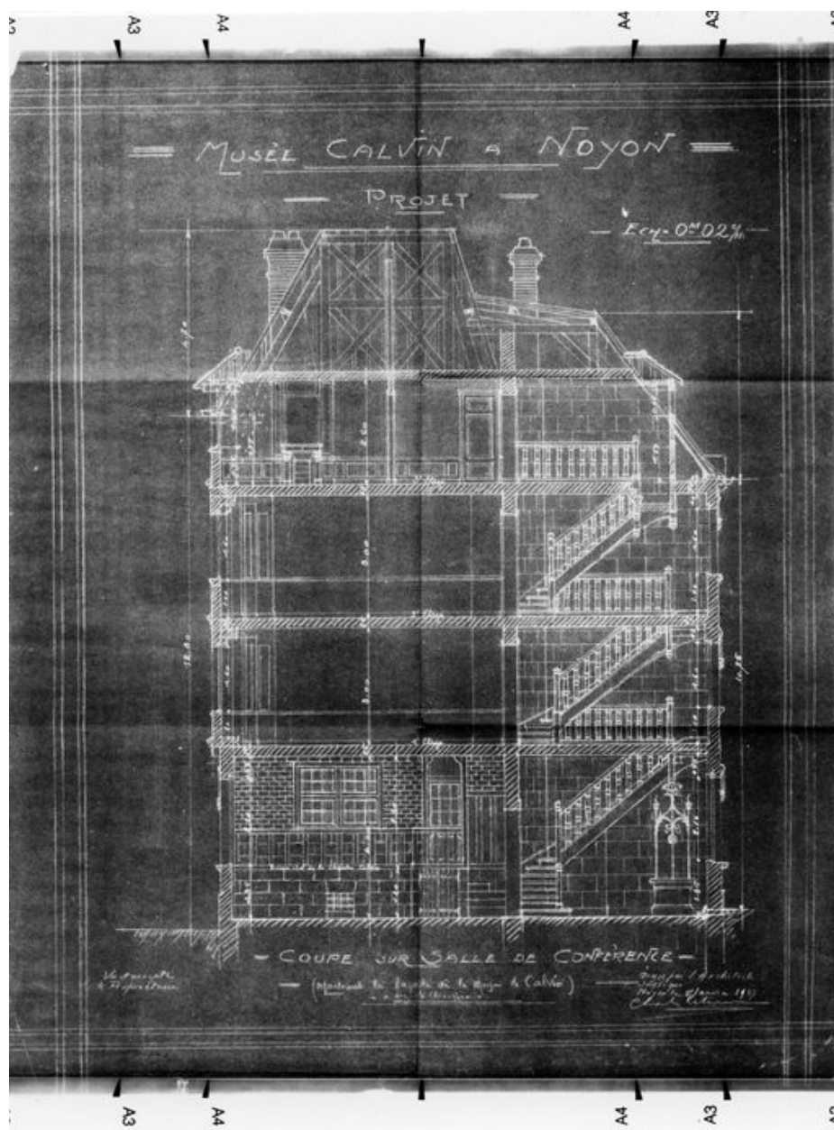
Coupe sur la salle de conférence. Projet de restauration, par Letrosne, 1927 (AC Noyon).
