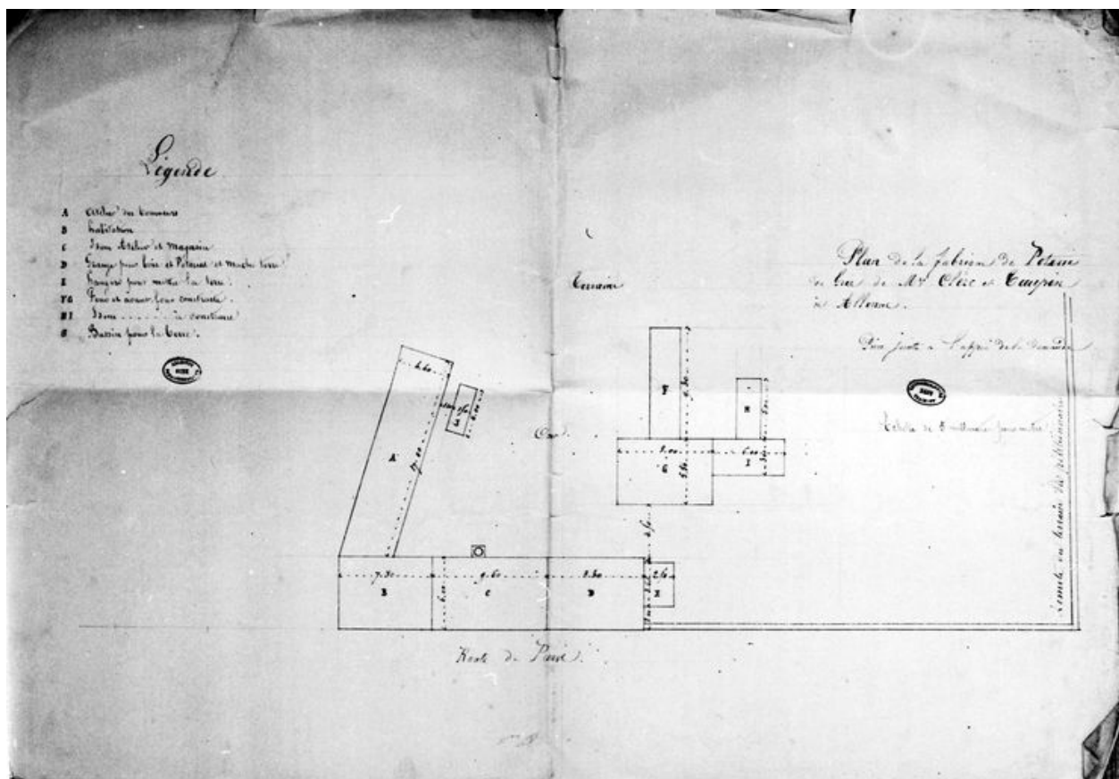
Plan de la fabrique Clerc et Taupin à Allonne, 1850 (AD Oise, MP241).
