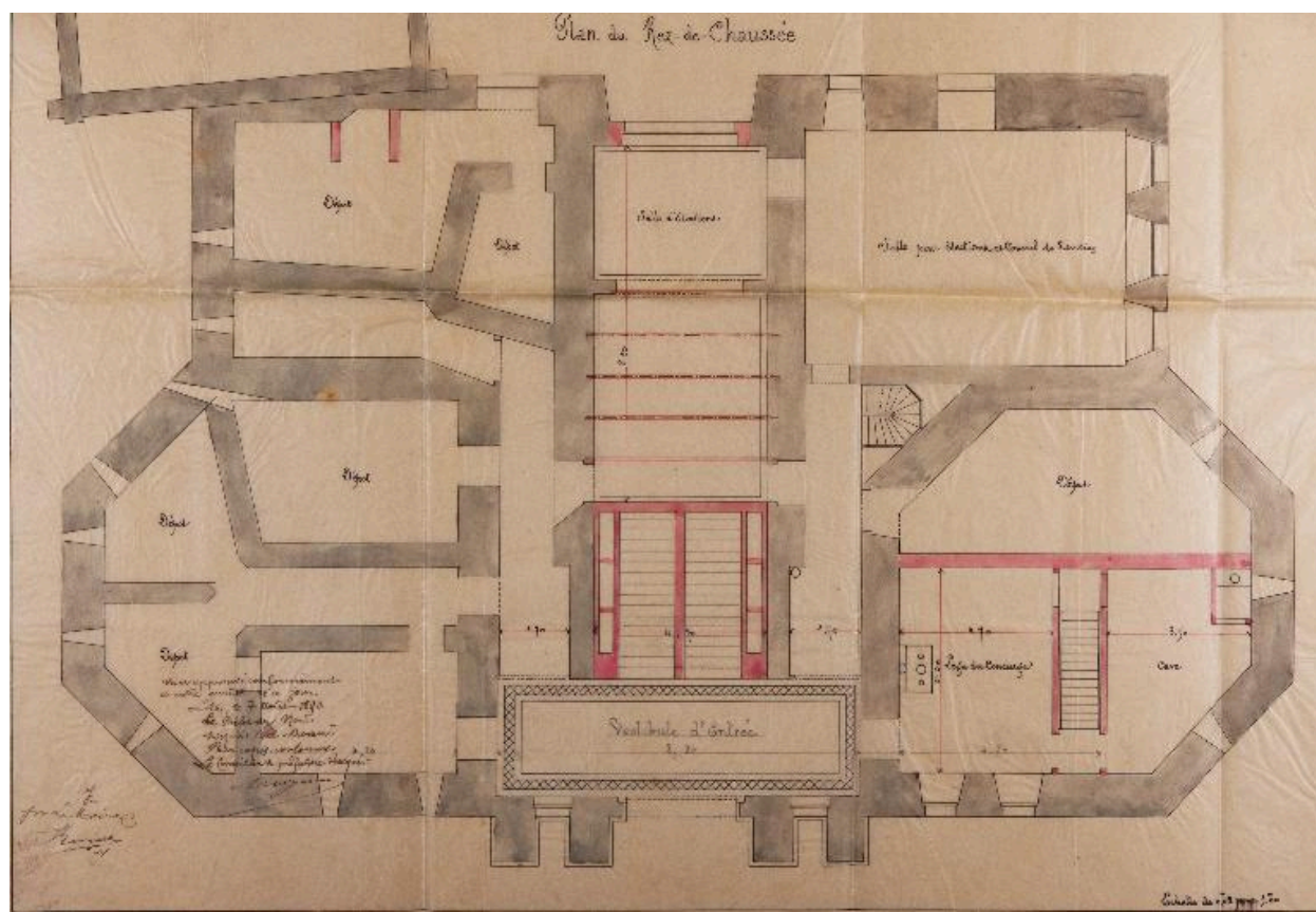
Plan du rez-de-chaussée (correspondant à la cave), Vandembuleke (?) architecte, 1890 (AD Nord, Série 2O 525/87).
