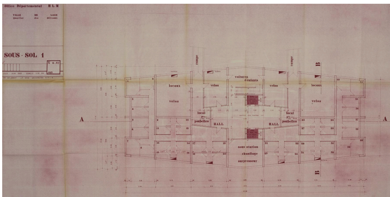
Plan du premier sous-sol de la tour Kennedy, juin 1963, F.-P. Delannoy et J.-P. Secq (arch.) (AD 59 ; 1465 W 66).
