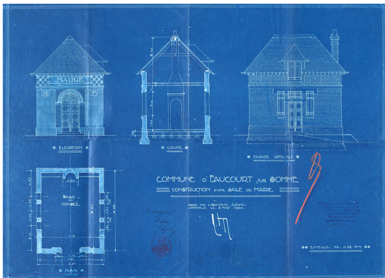
Plan et élévation pour la construction d'une salle de mairie, par Marcel Dingeon, 2 mars 1924 (AD Somme ; 99 O 1483).
