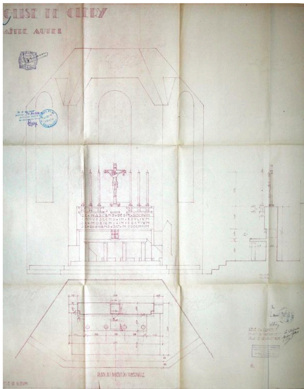
Maître-autel (plan, coupe et élévation au niveau du tabernacle), Jacques Debat-Ponsan (architecte), 24 juillet 1931 (AD Somme ; 99 O 1182).
