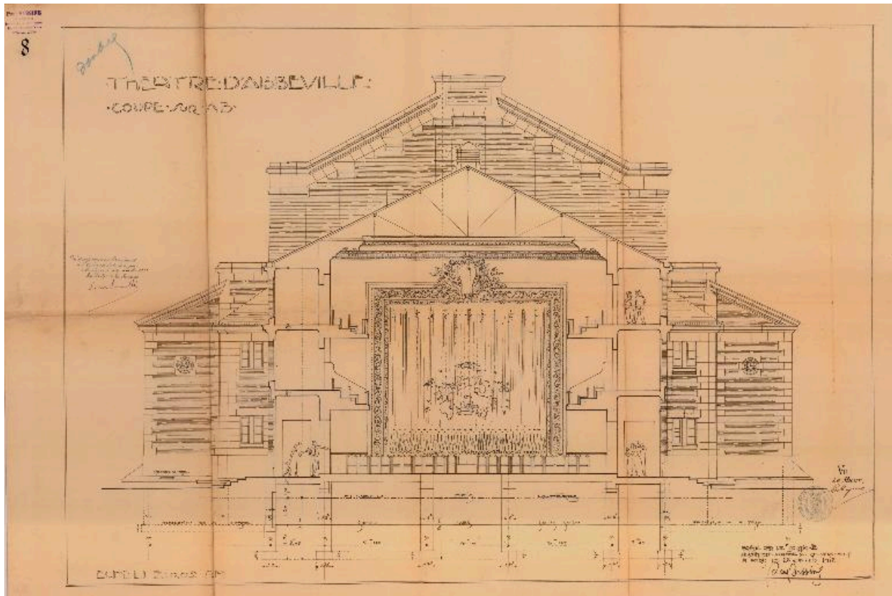
Coupe transversale, tirage, par Paul Bessine, 25 janvier 1912 (AD Somme ; 99 O 35).
