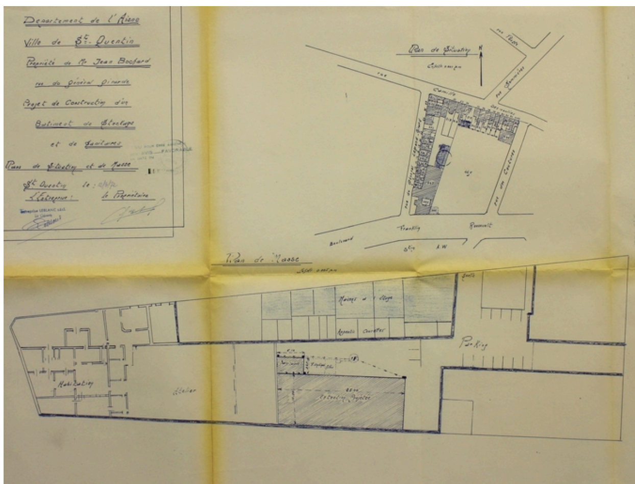
Plans de situation et de masse comportant le projet d'extension des ateliers en 1972 (AC Saint-Quentin).
