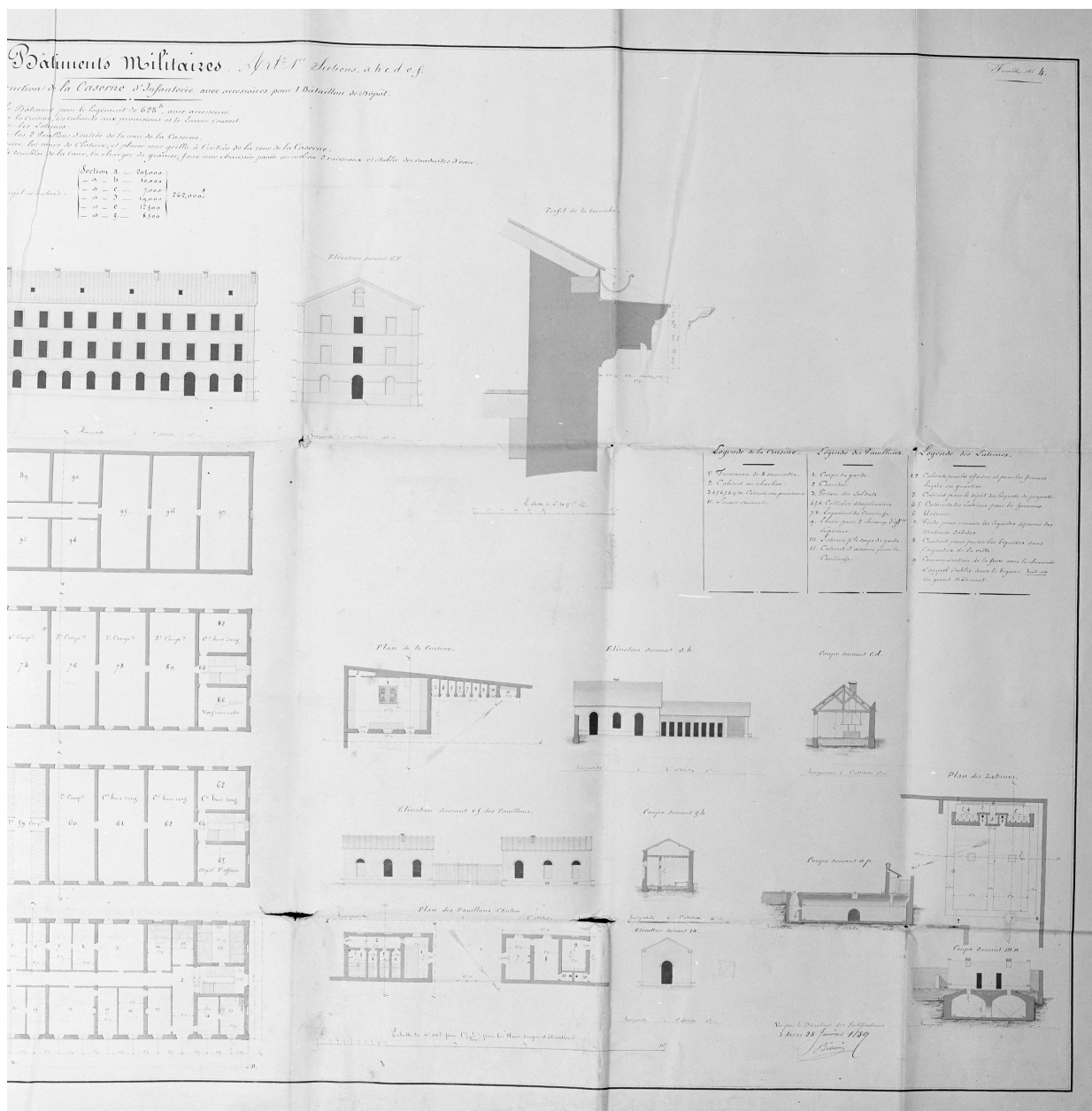
Pavillons d'entrée, cuisine : plans, coupes, façade, 1859. A. Génie Vincennes, Boulogne, art. 8, section 1, carton 9.
