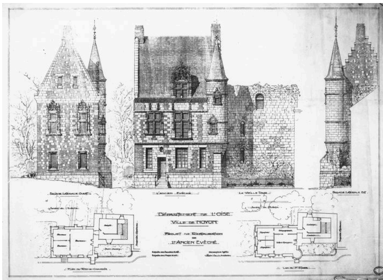
Plans et élévations de la tour du 12e siècle et de l'aile du 16e siècle. Projet de restauration par Collin, 1923.
