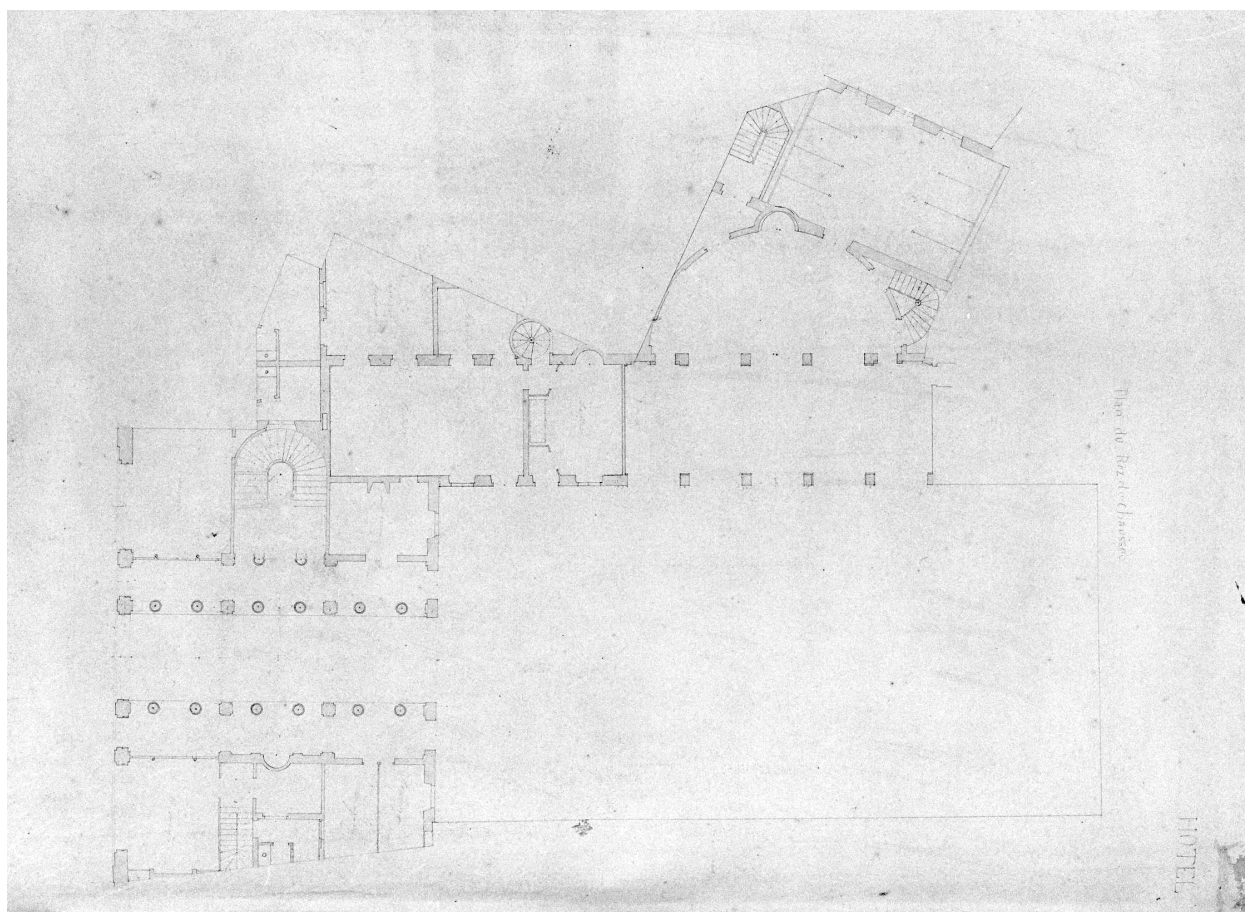
Plan du rez-de-chaussée. B.M. Boulogne-sur-Mer, mss. 535 P, pl. 100.
