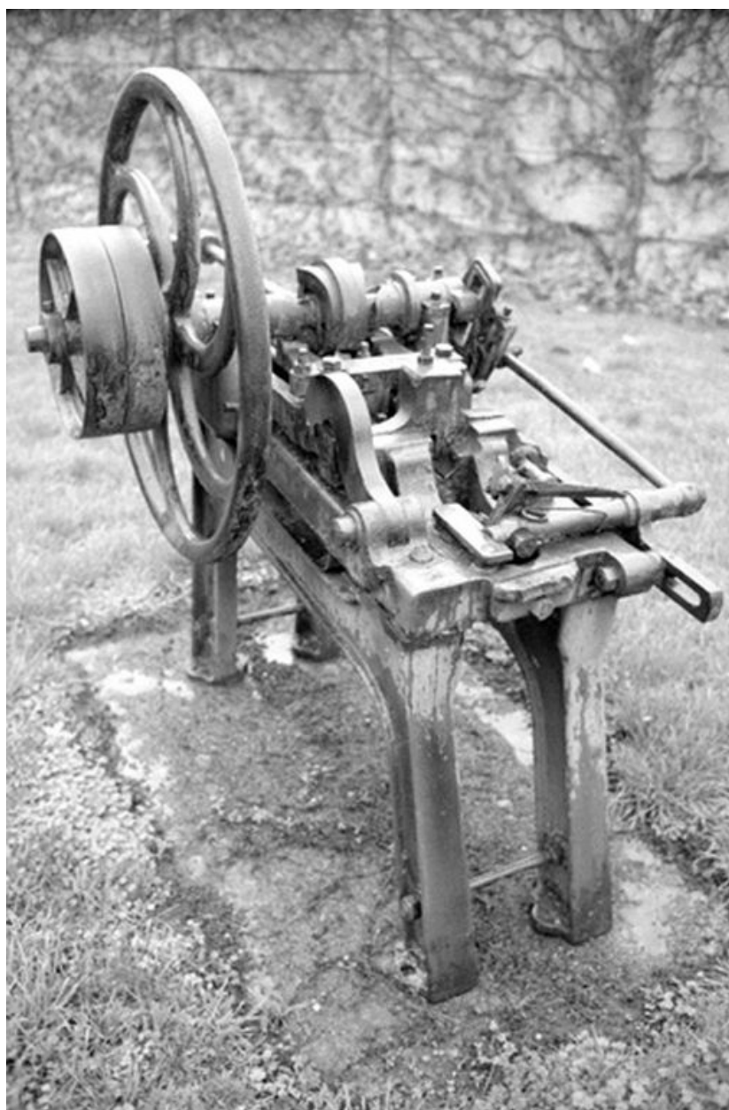
Machine à ouvrir les clous.
