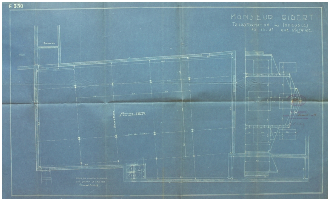
Plan de l'atelier construit en 1923, par Brassart-Mariage (AC Saint-Quentin).
