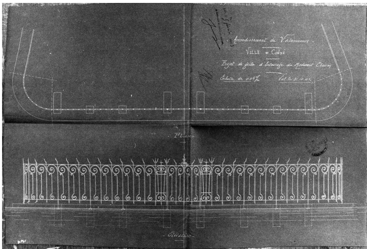
Projet de grille de clôture (non retenu), plan et élévation partiels, 1902 (AD Nord).
