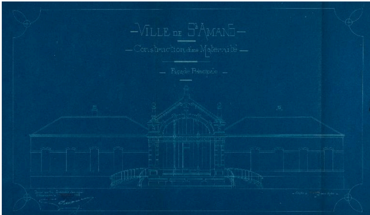
Projet de maternité, élévation antérieure, Gustave Dupont architecte, 1903 (AH, centre hospitalier de Saint-Amand-les-Eaux).
