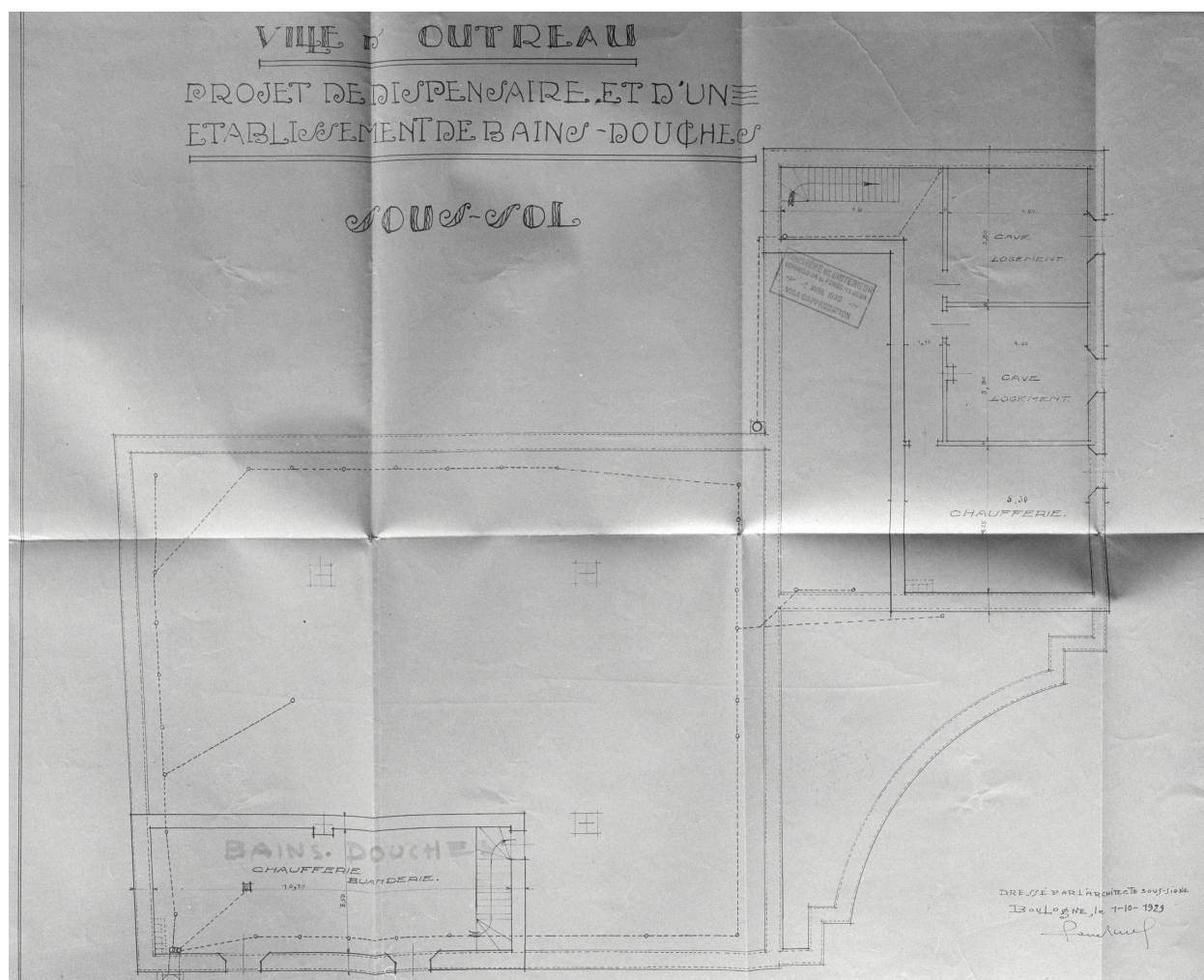
Plan du sous-sol (AD Pas-de-Calais, 20, n° 23).
