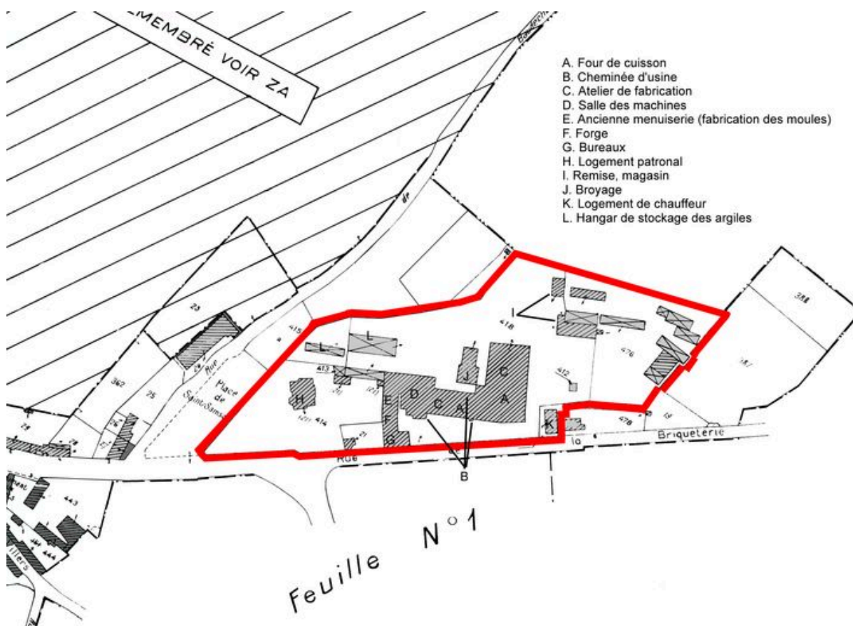
Plan masse détaillé de l'usine, extrait du plan cadastral de la commune, section A1, 1985, éch : 1/1250e.
