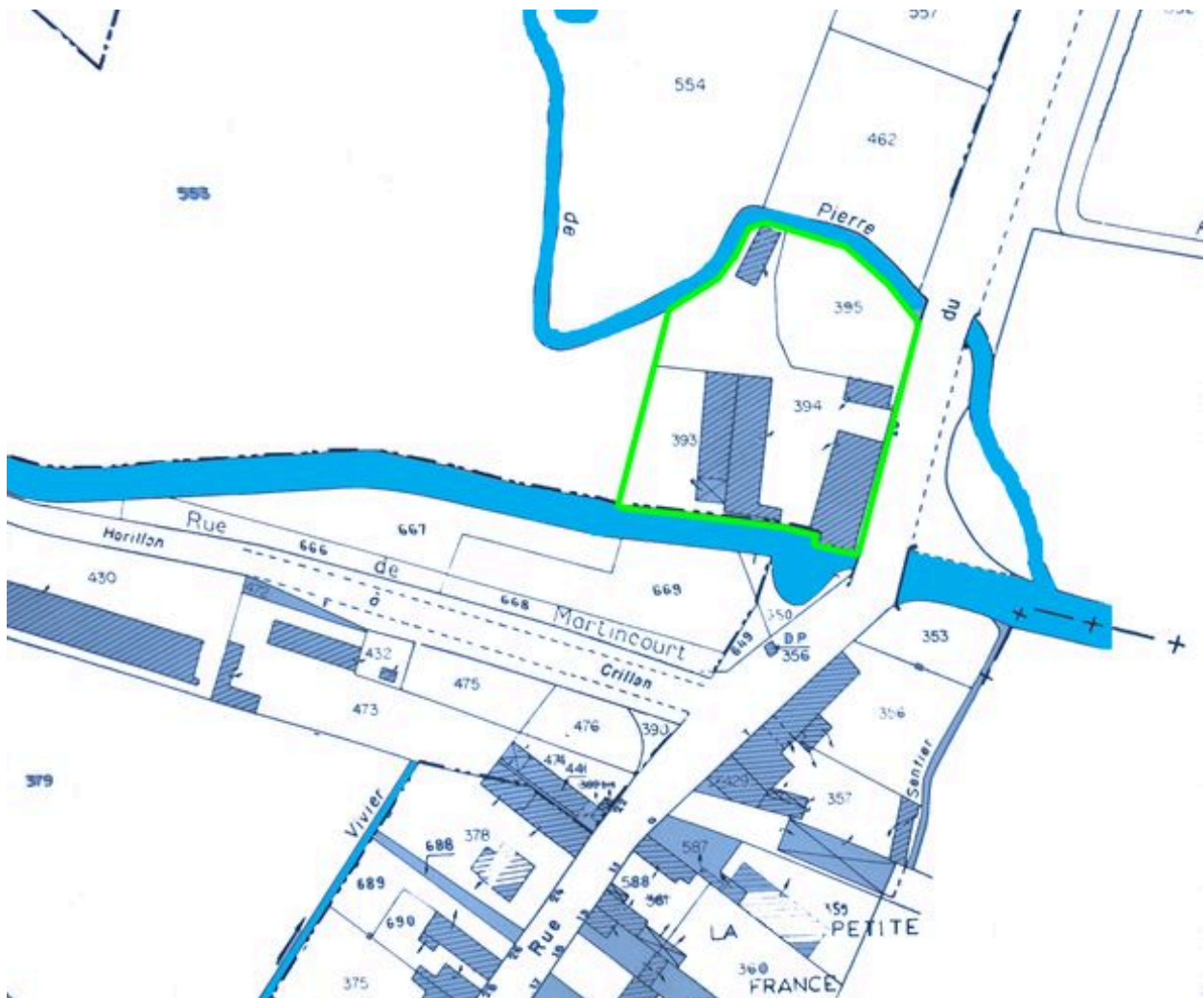
Plan masse de la minoterie, extrait du plan cadastral de la commune de Crillon, section C, 1983.
