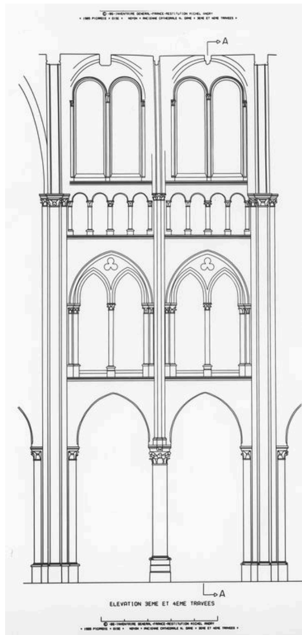
Elévation nord (3e et 4e travées de la nef).
