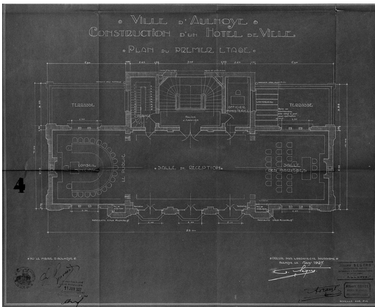
Plan du premier étage par Joseph Ségers et Albert Rouzé, architectes, mars 1927 (AD Nord ; O33/86).
