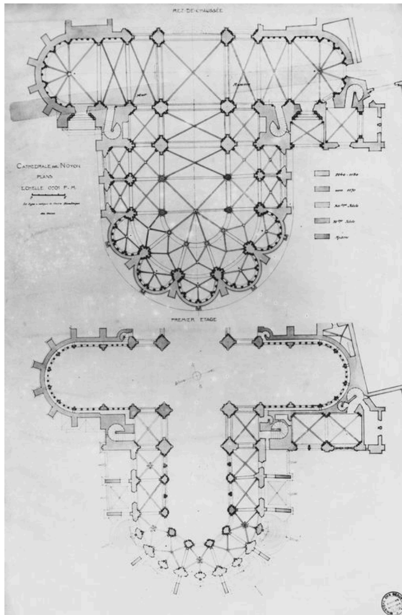
Plan du chœur et du transept, par Barbier, 1925.
