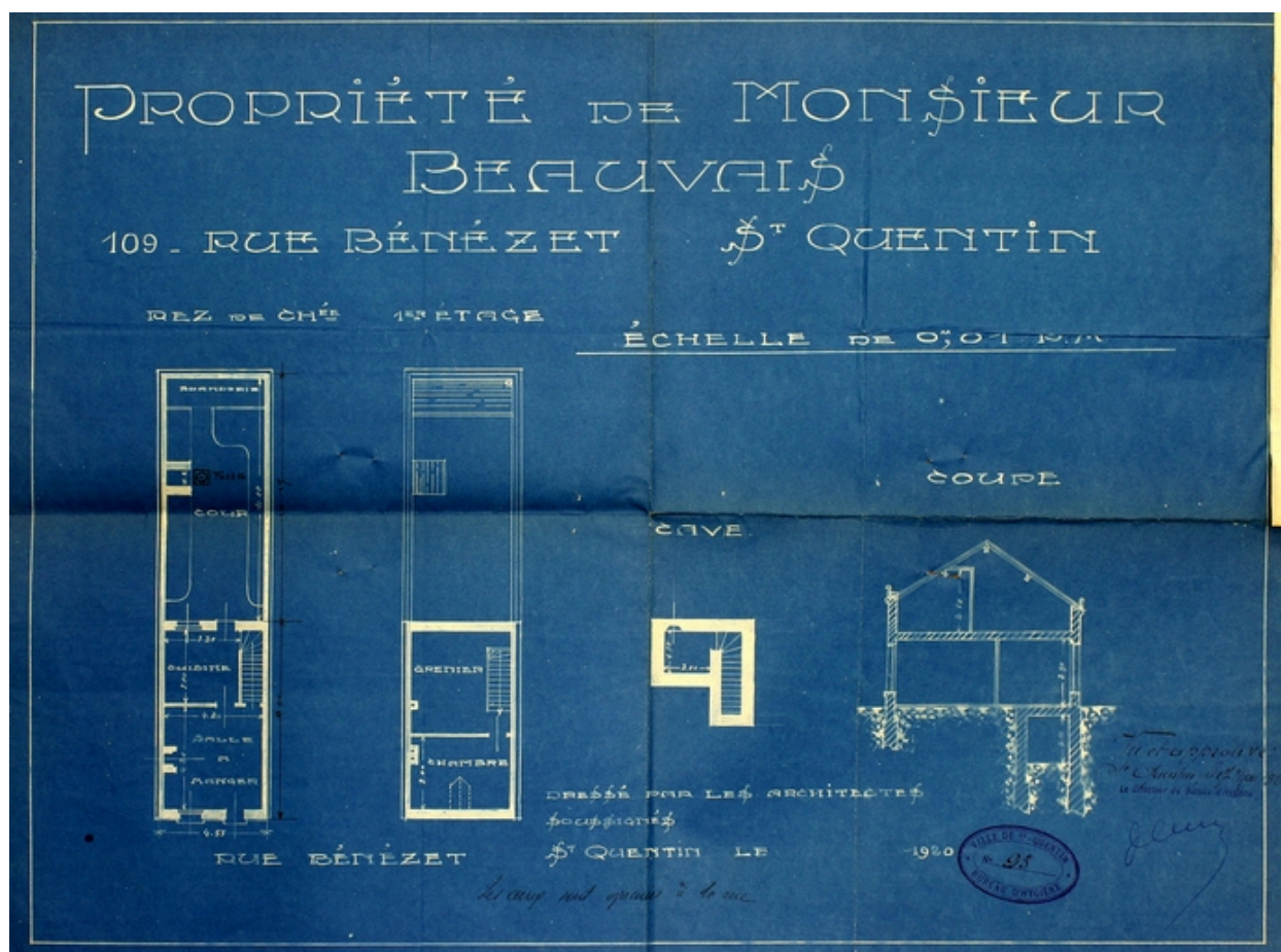
Plans d'une maison ouvrière de la rue Bénézet, 1920 (AC Saint-Quentin).
