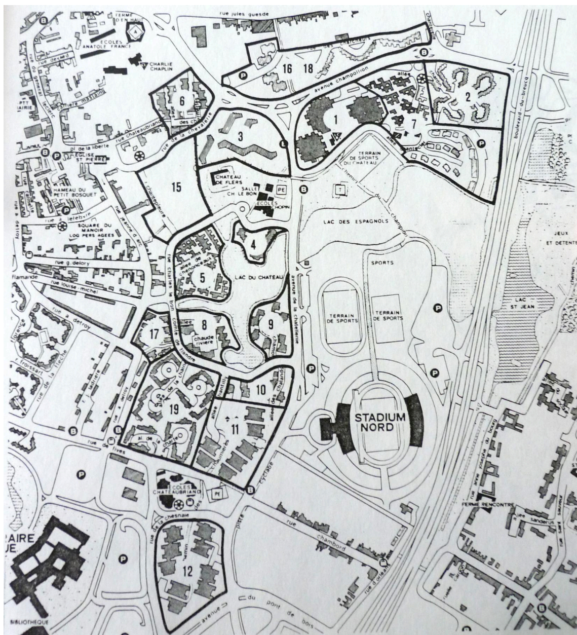
Plan d'implantation des îlots d'habitation du quartier Le Château en 1981, d'après La Population nouvelle, études 78, 79, 81, E.P.A.L.E., Etudes et documents, 1982 (AC Villeneuve d'Ascq, salle de consultation).
