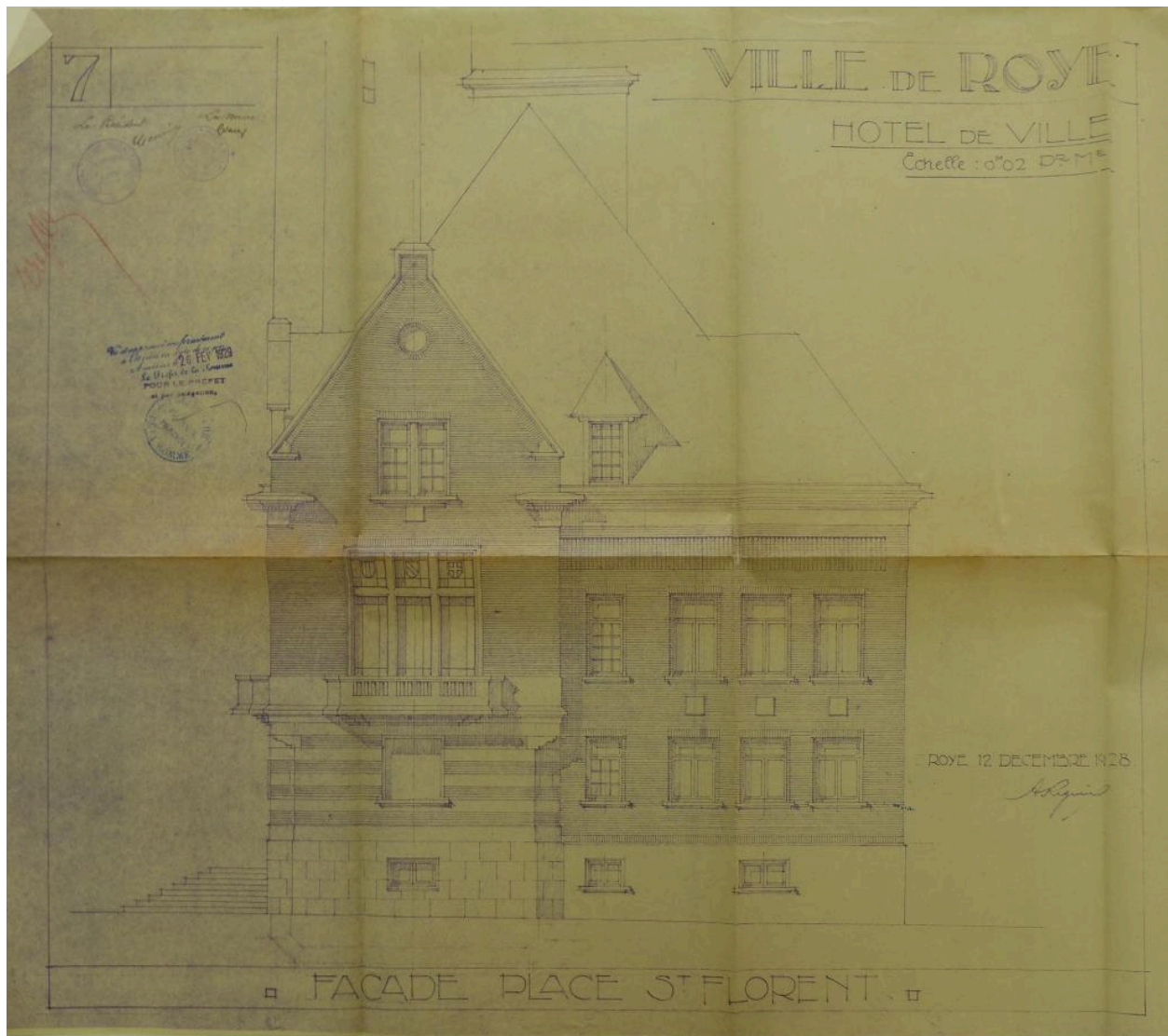
Ville de Roye. Hôtel de ville. Façade place Saint-Florent. A. Régnier architecte, 1928 (AD Somme ; 99O 3296).
