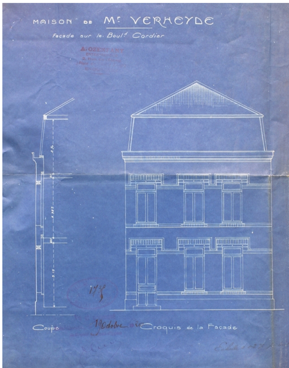
Façade antérieure de l'habitation et des bureaux, par Ozenfant, 1920 (AC Saint-Quenin).
