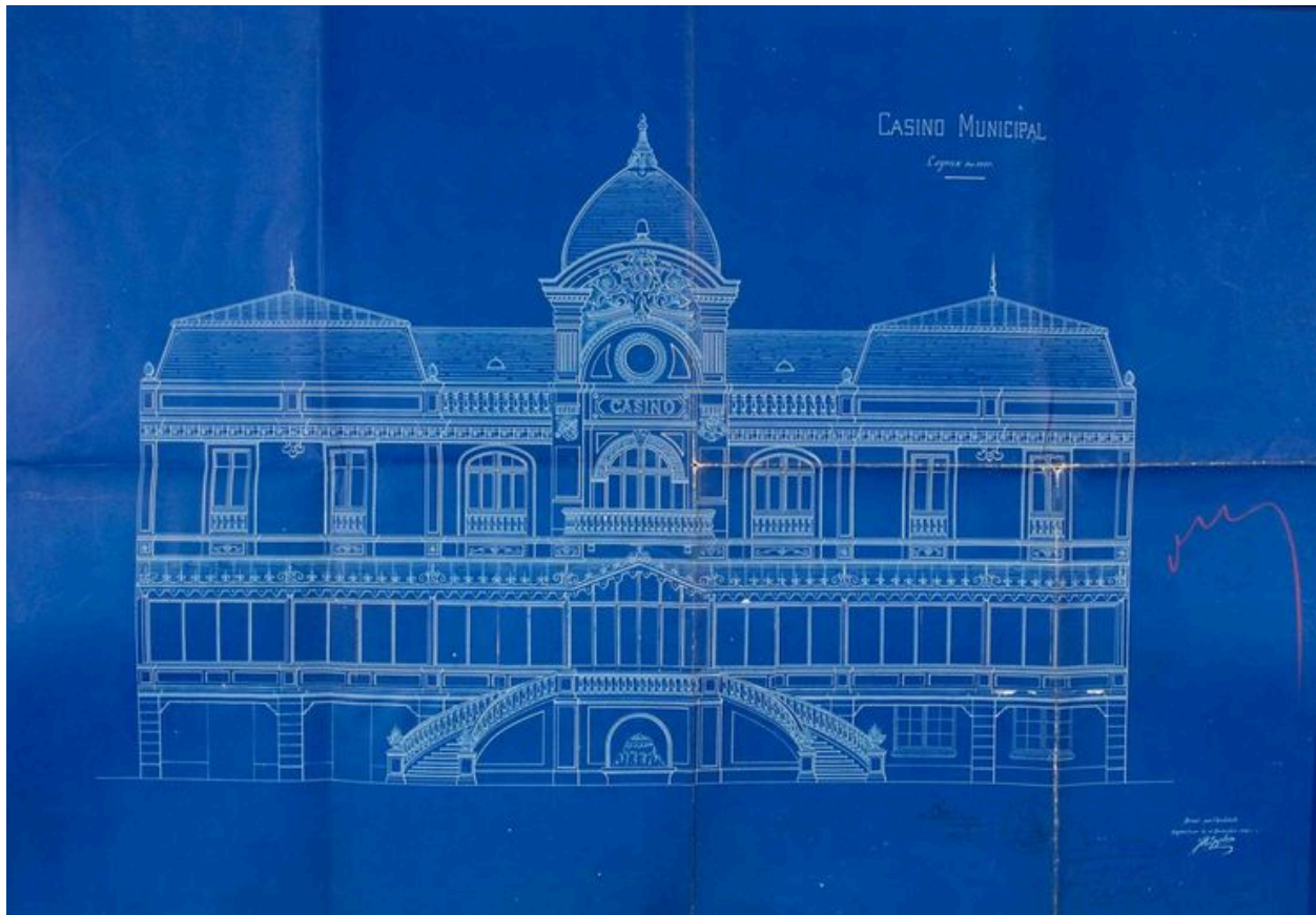
2e casino de Cayeux-sur-Mer, élévation sur mer, par Léon Kämpfer architecte, 1908 (AD Somme).
