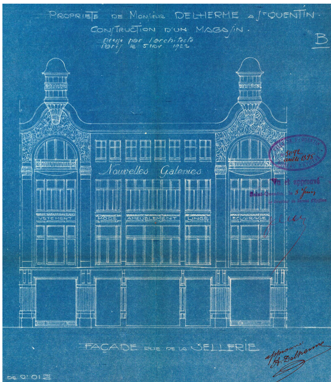
Élévation de la façade nord, rue de la Sellerie, 5 novembre 1922 (Archives municipales de Saint-Quentin).
