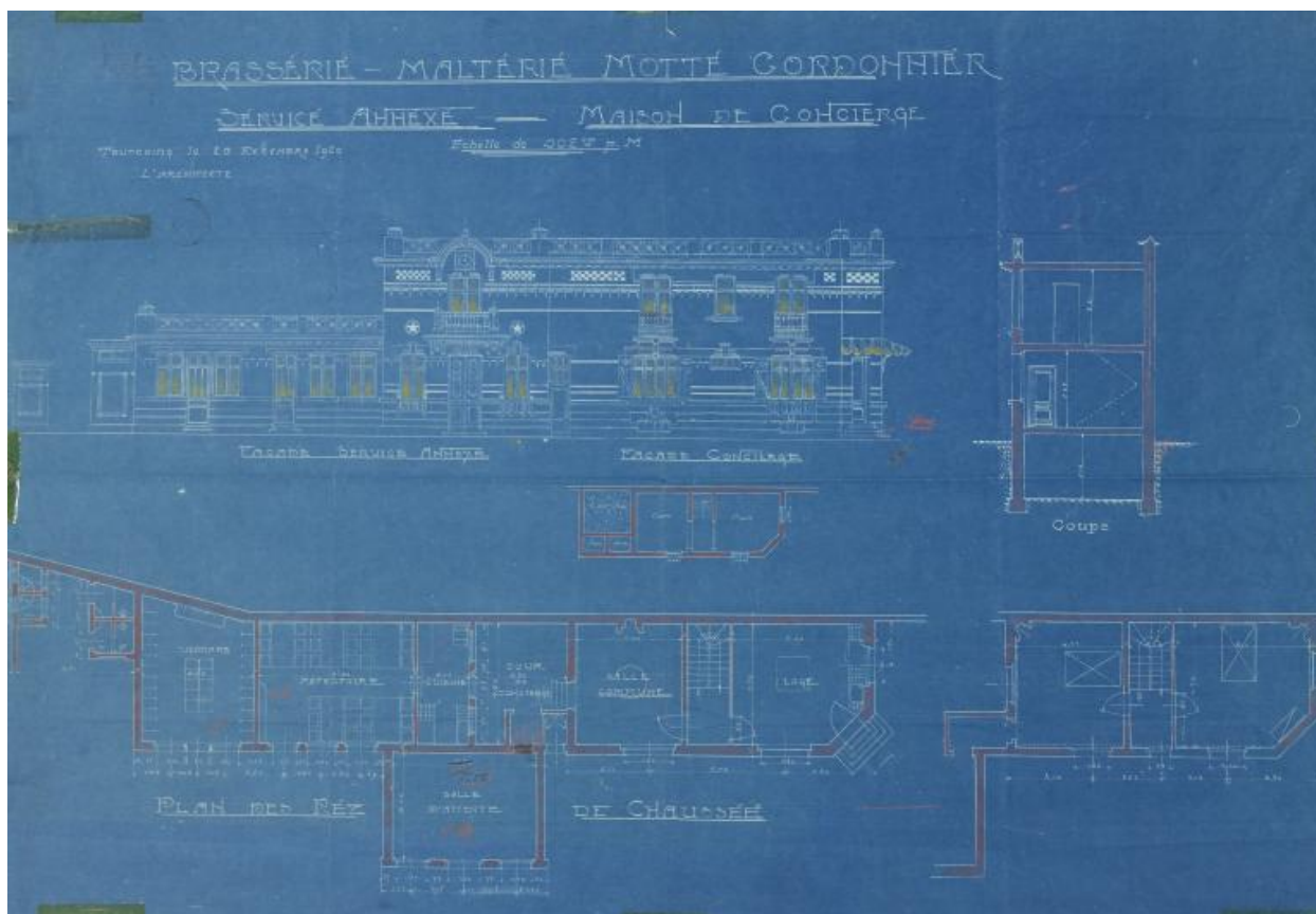
Brasserie-malterie Motte-Cordonnier. Service annexe. Maison de concierge. Coupes, élévation. Plan de l'architecte Georges Forest, 20 décembre 1920 (coll. part. Motte).
