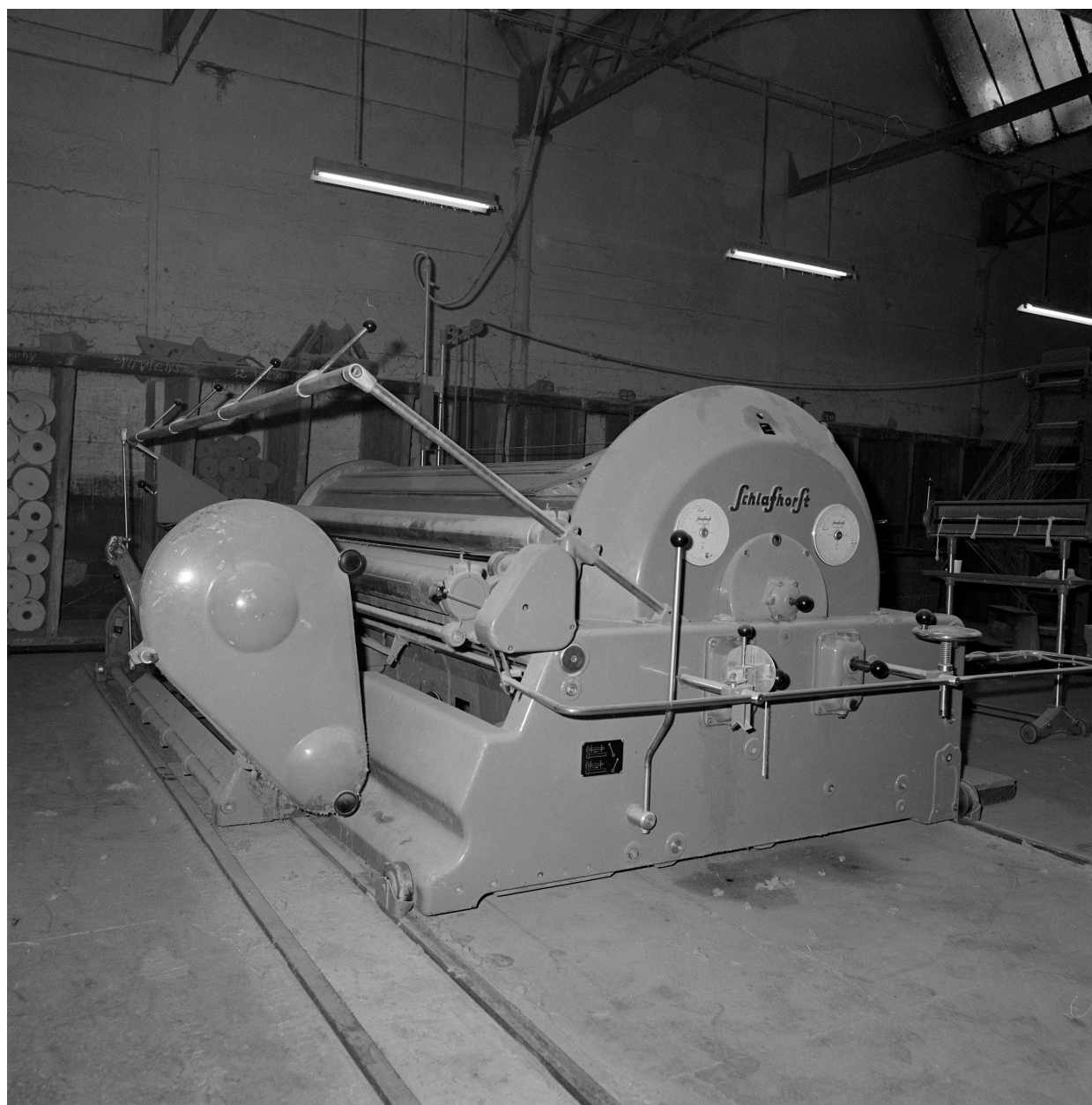
Poste d'ourdissage sectoriel et d'ensouplage (Schlafhorst, RDA).
