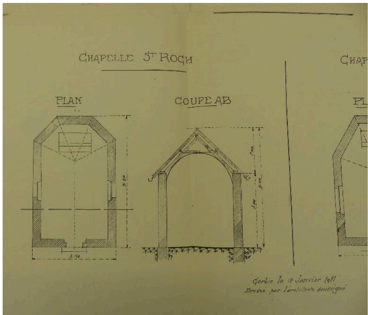
Plan et coupe de la chapelle Saint-Roch du Hamel, 1921 (AD Somme ; 10R 628).
